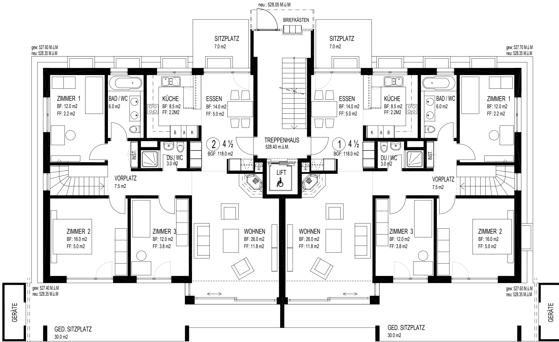
ERDGESCHOSS HAUS A M. 1:100 / 30.01.2006
